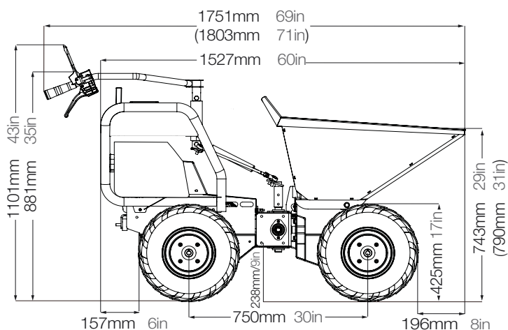
Dimensioner B300 (B450)
